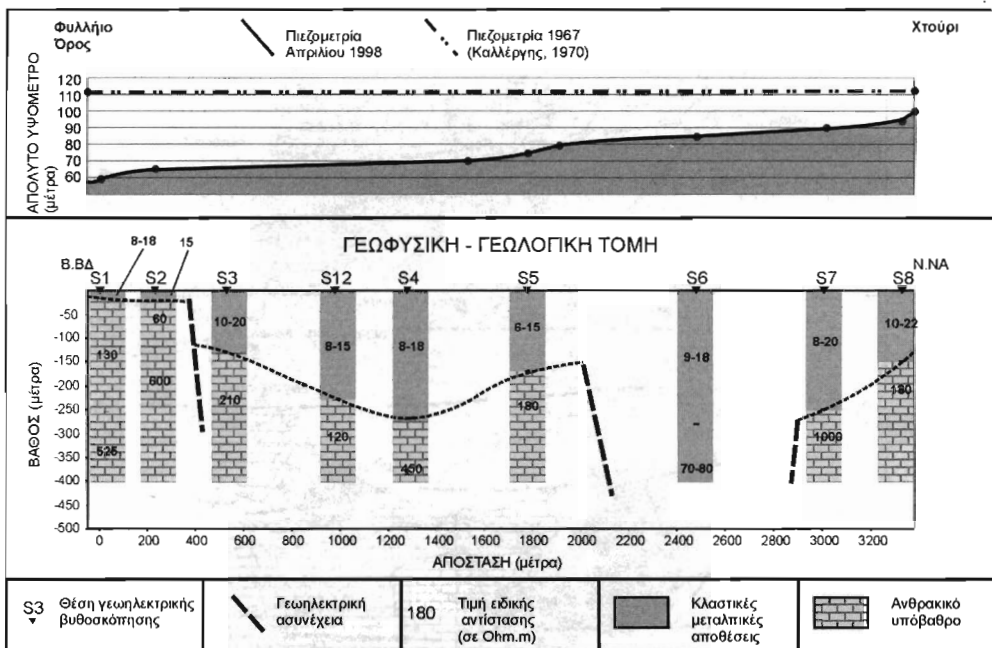
Εικόνα 3: Συγκριτική τομή της ερμηνείας των γεωηλεκτρικών διασκοπήσεων (κάτω) και της μεταβολής της στάθμης της υδροφορίας στην ίδια περιοχή από το 1967 ως το 1998.
