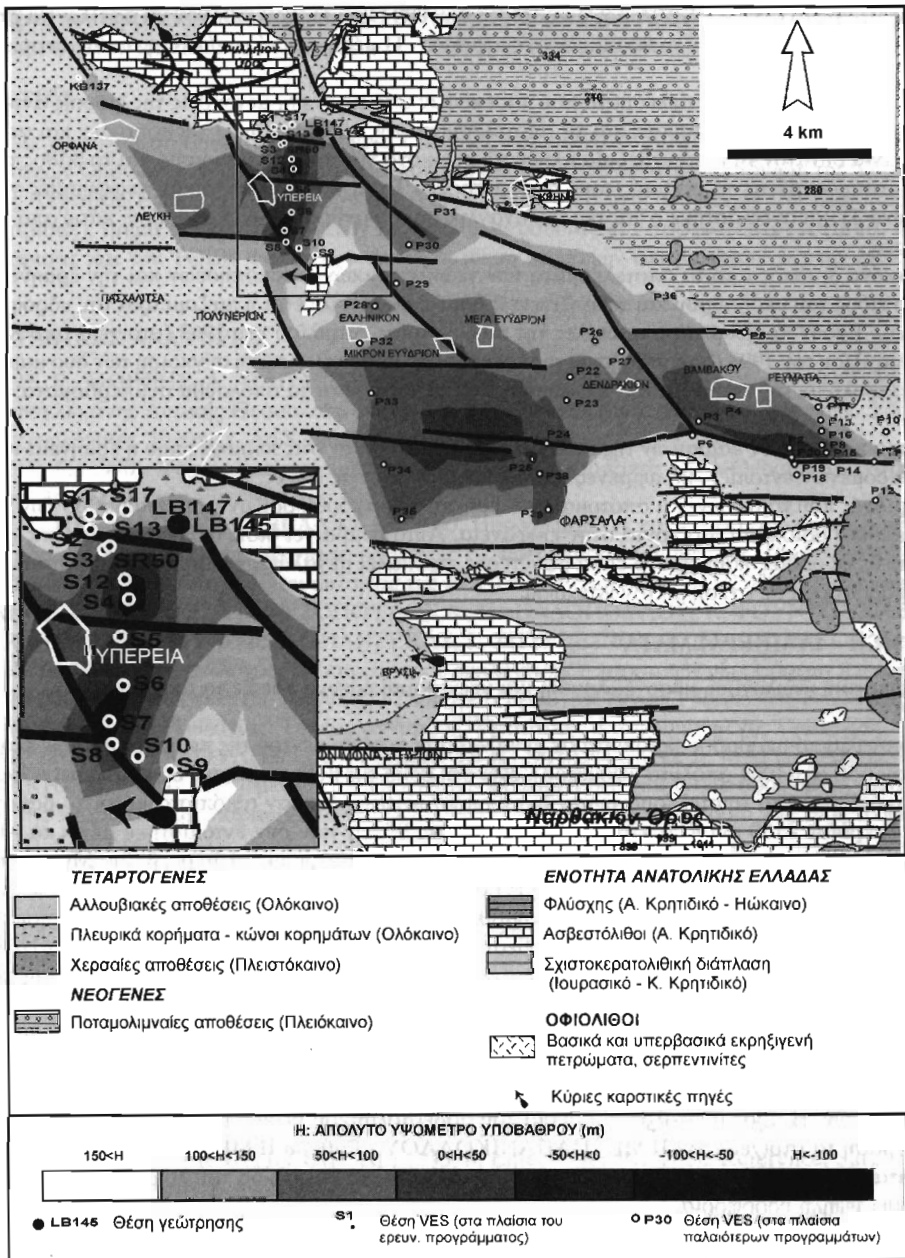
Εικόνα 4: Υπεδαφικός τεκτονικός χάρτης με τα σημεία διακοπήσεων.
